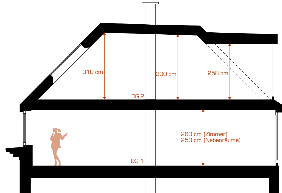
Schnitt 1
