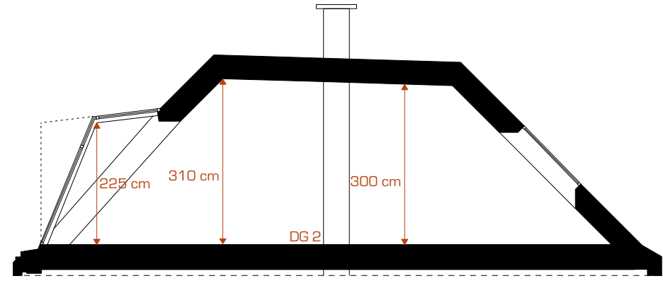
Schnitt 2
